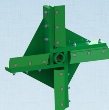
OPCIONAL - 4 FACAS ROTOR EC - 4.000 / 4.800 ECT- 4.000/ 4.800 PLUS ECTR - 4.000/ 4.800 PLUS
